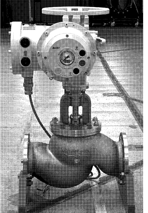
船舶向けなどで採用を目指す水素防炎仕様のバルブアクチュエーター(写真上部)
