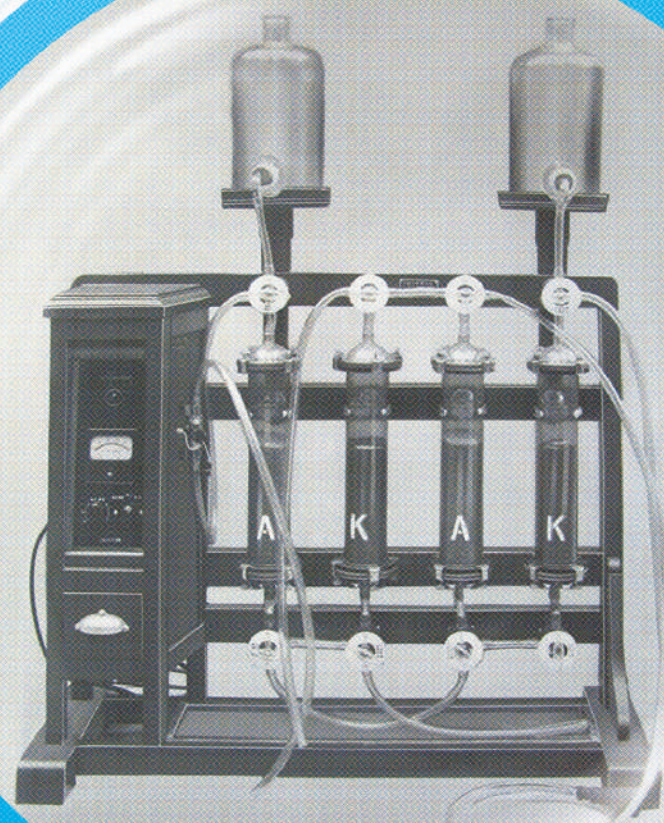
無熱蒸溜水製造装置
