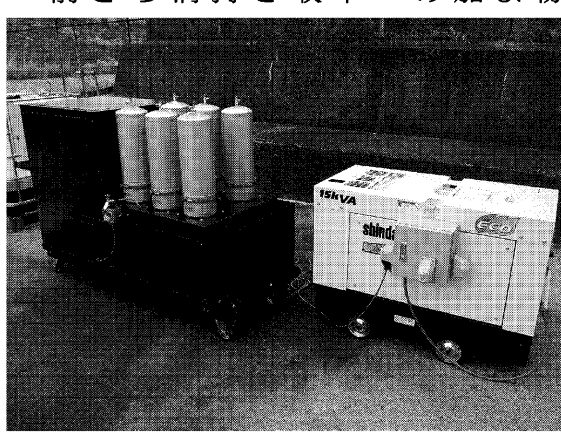
工場を電源を使用せず自前の発電機で再生装置を稼働する 三重県桑名市中央町3丁目66番地 TEL.0594-22-4521 FAX.0594-22-4523 https://www.nayaden.co.jp/
