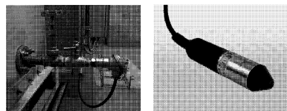
横付水位センサー 投入式水位センサー
