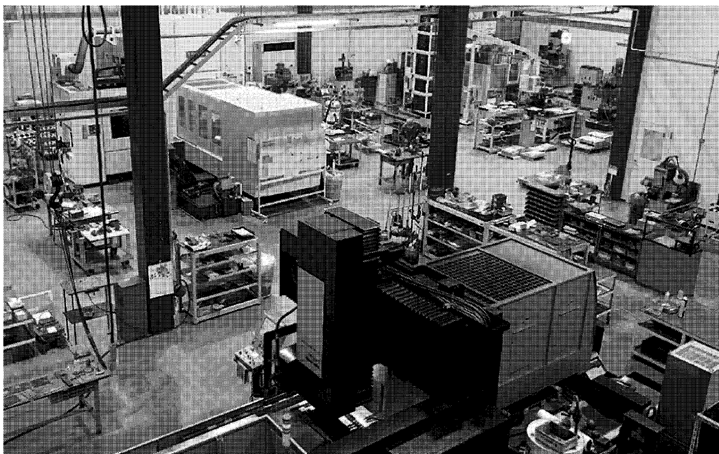
城山産業のモーターコアの加工ライン
