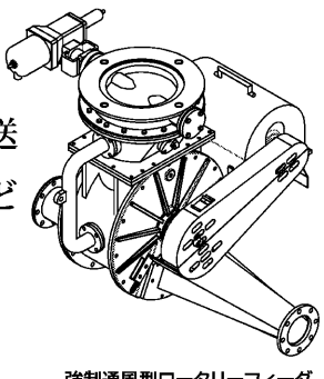
強制通風型ロータリーフィーダ
