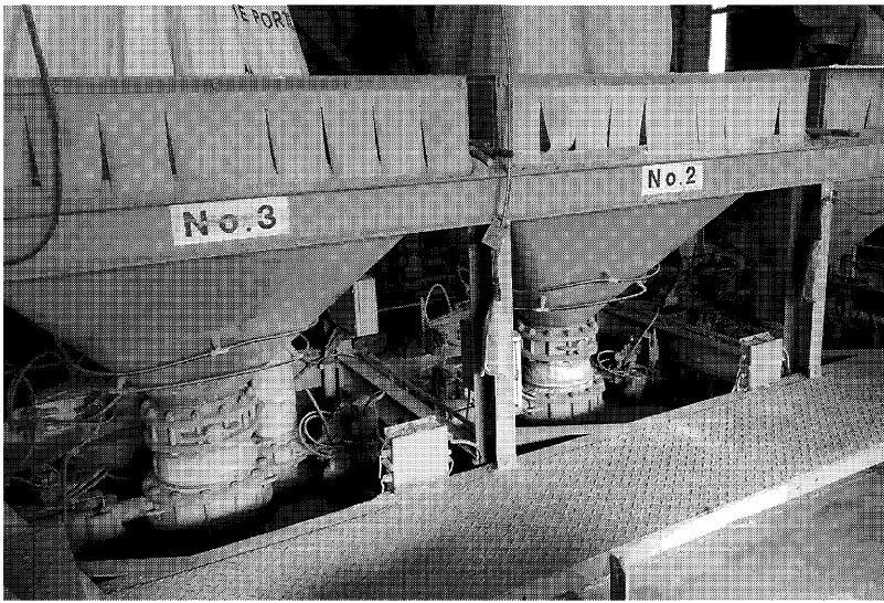
いろいろな粉体を一つの輸送機で計量して送る装置
