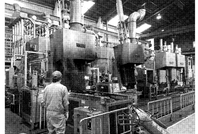
日高工業の本社工場の既存熱処理ライン
