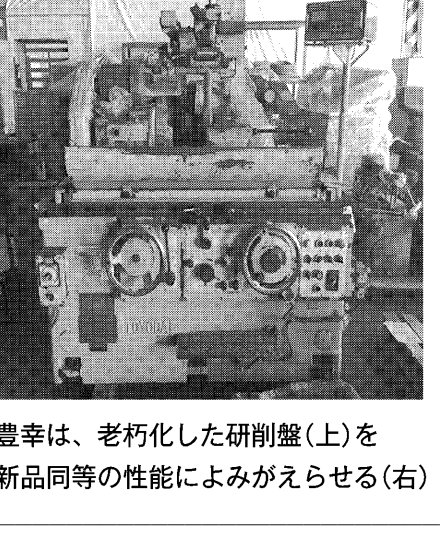
豊幸は、老朽化した研削盤(上)を新品同等の性能にのみがえらせる(右)
