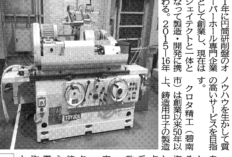
豊幸は、老朽化した研削盤(上)を新品同等の性能にのみがえらせる(右)
