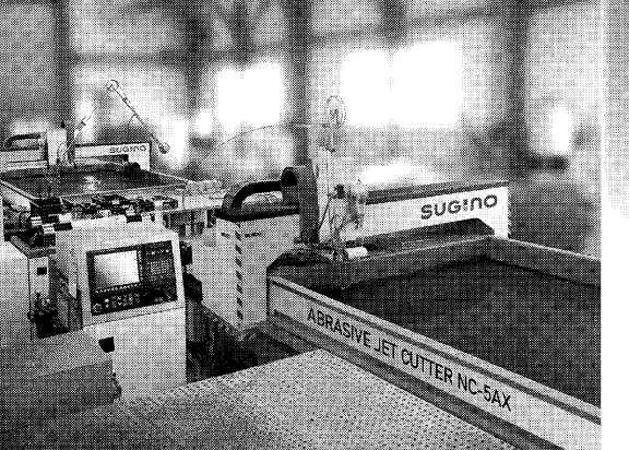
ウォータージェット切断機 280t×2000×4000
