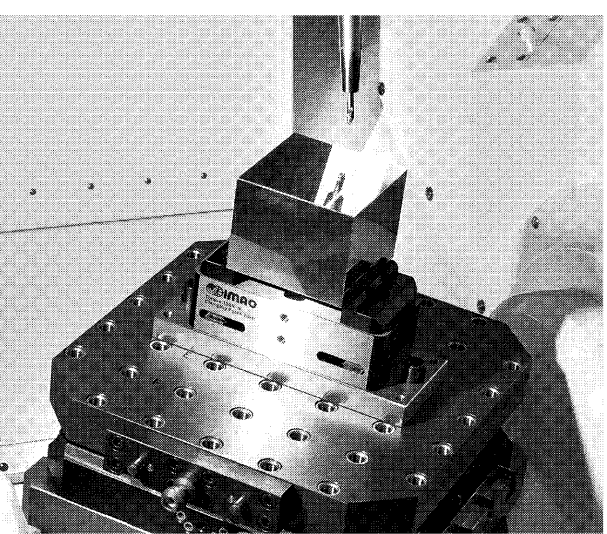
クランプユニットを投入(イマコーポレーション)
