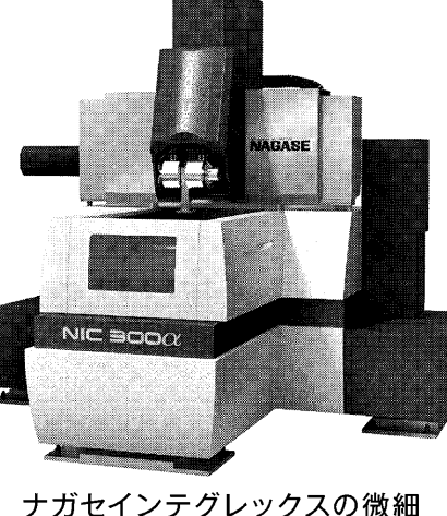
ナガセインテグレックスの微細形状加工機「NIC-300a」
