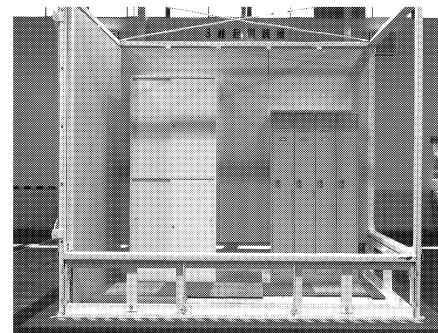
阪神大震災（JMA神戸波）による耐震性能実証済み ※株式会社ワコー（パレット振動実験室にて）
