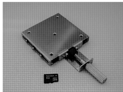
薄型・軽量 板金製Xステージ
