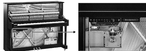
電子音の信号を振動に変えるトランスデューサー
