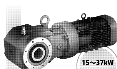
ベベル・パディボックス® 5シリーズ 0.75~37kW
