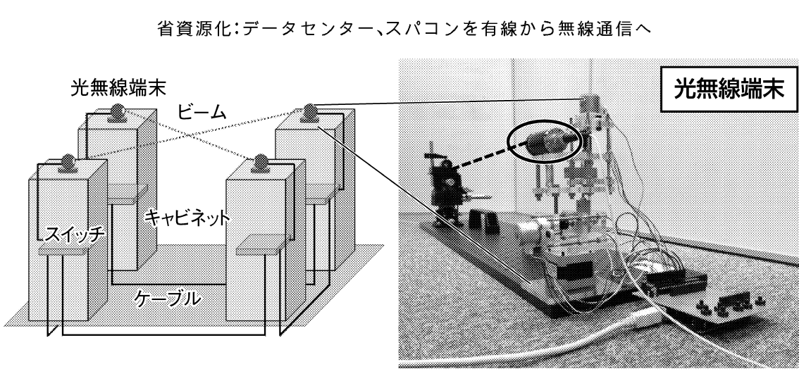
図2 毎秒40ギガビット光無線リンクを用いたスパコン、データセンターネットワークの試作と構想(鯉渕研究室)
