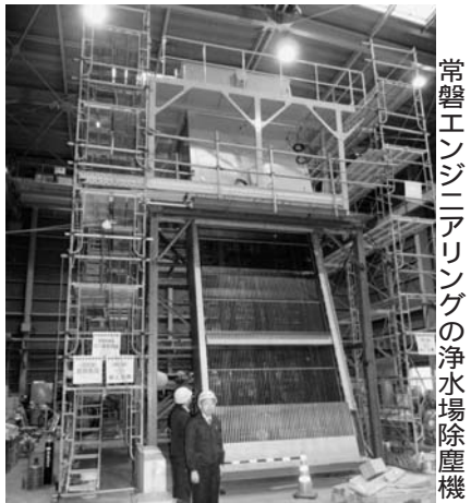
常磐エンジニアリングの浄水場除塵機
