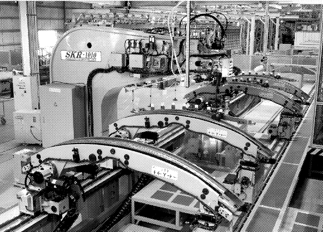
スギヤマメカトロのオートマチックリベッター
