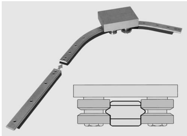
直線、曲線レールとも安定走行可能な独自仕様のベアリング機構を採用
