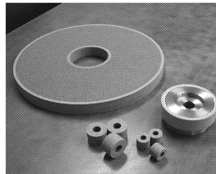
トパーズ砥石(黄色系ビトリファイド)CBN砥石
