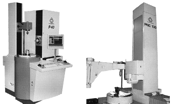
クリンゲルベルグ社製(P40)型 三次元測定・ナリ測定を実現 クリンゲルベルグ社製(PNC130VA) 最大径1,300mmインターナルギヤー(要相談)
