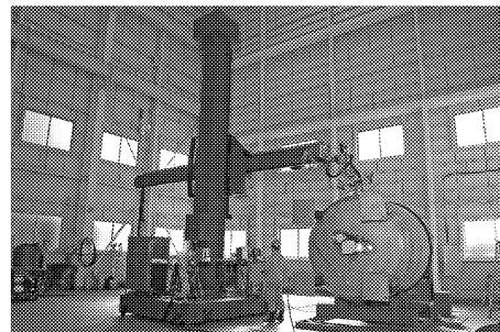
大型プラズマ溶接機
