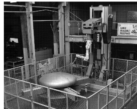
鏡板軍曹・穴あけ・開先切断ロボット
