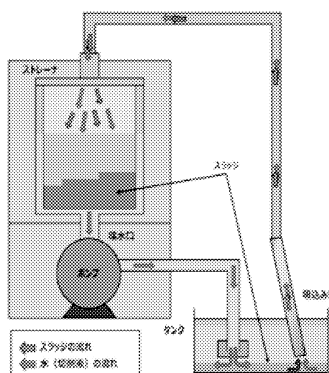
スラッジ回収装置のしくみ
