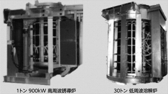
1トン 900kW 高周波誘導炉
