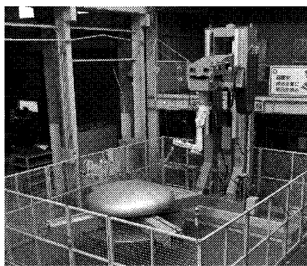
鏡板野書・穴あけ・開先切断ロボット
