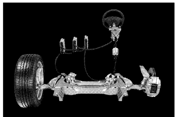
協和工業のステアリングジョイントとシャフトが採用された日産の次世代ステアリングシステム
