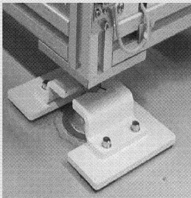
▲ 工場:生産設備使用例 PAT.P
