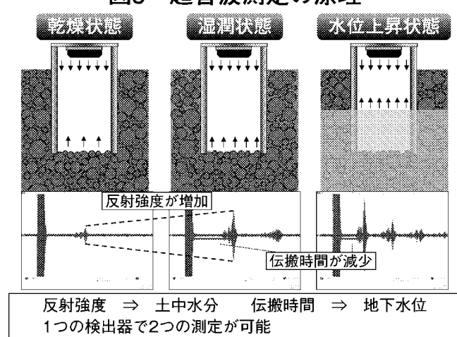
図3 超音波測定の原理
