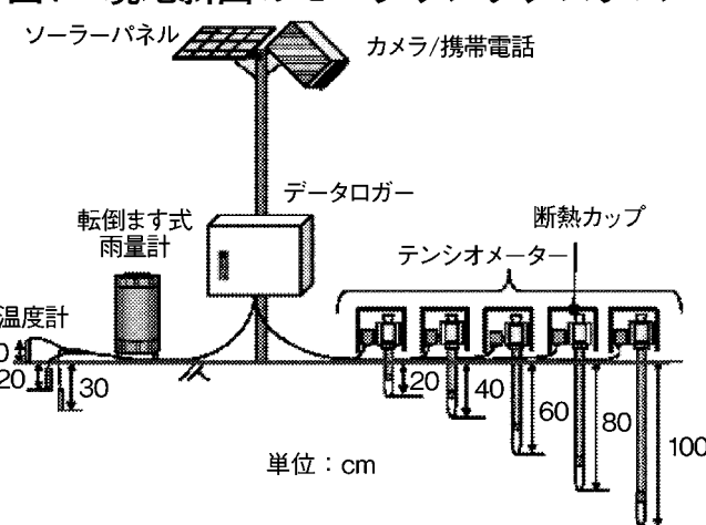
図1 現地斜面のモニタリングシステム
