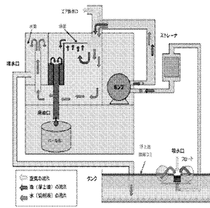
浮遊油回収装置 油水分離のしくみ
