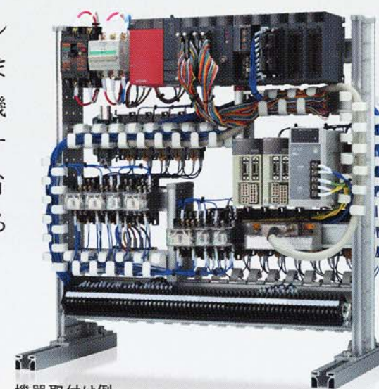
機器取付け例
