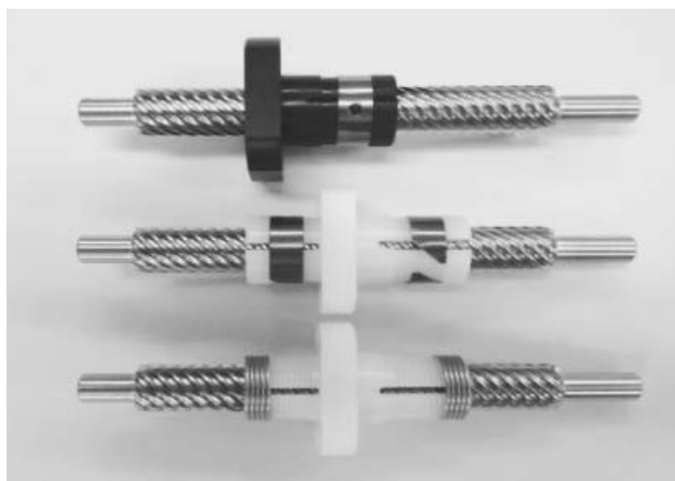
「グリップネジ」の板バネ式④、コーイルバネ式⑤は摩擦が進行してもテーパネジの長さ分、何度でも調整できる
