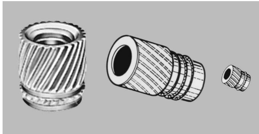
「SECCAMのインサート」は熱や超音波を使わずに成形品に圧入でき、作業の効率化が図れる
