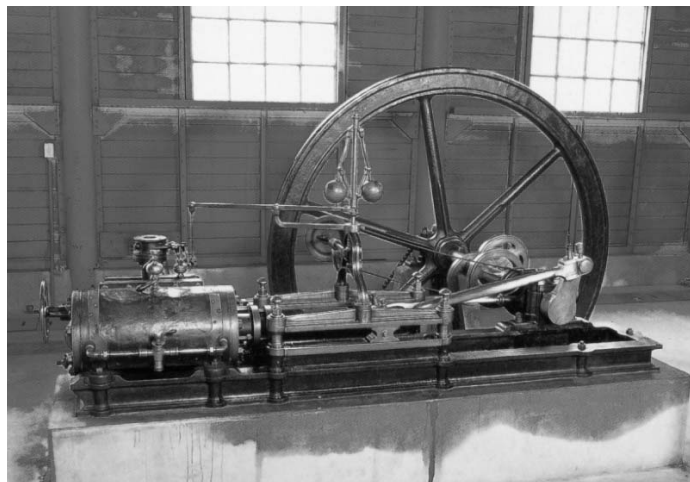
復元を目指す「プリュナエンジン」
