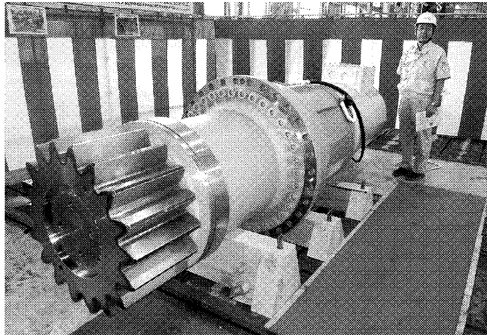
神鋼造機の世界最大級のシールドマシン用減速機
