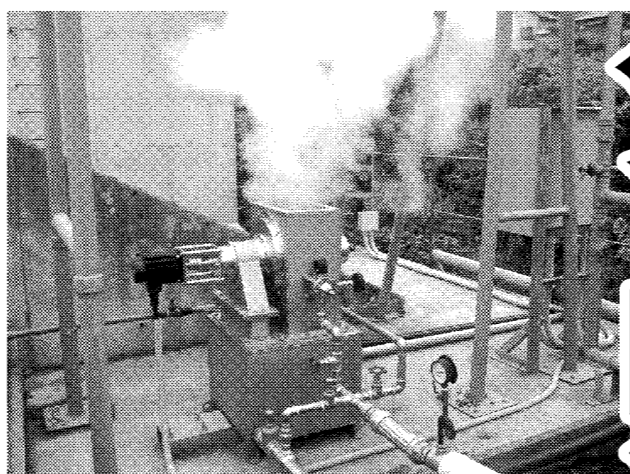
湯けむり発電装置 (大分県別府市)
