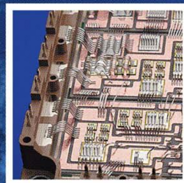
■デバイス技術 電気を無駄なく制御するIGBT パワー半導体
