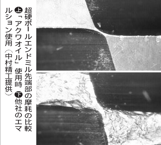
超硬ボールエンドミル先端部の摩耗の比較 ●「アクワオイル」使用時 ●他社のエマルジョン使用(中村精一提供)
