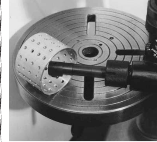
「インナーカットLG型」のカッターはネジ式で交換も簡単
