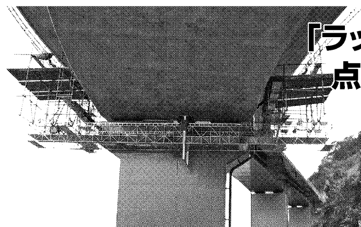
ラックレール式移動吊足場 ラック足場
