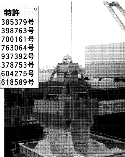
▲本船石炭揚荷役中12m3単索無線クラブ
