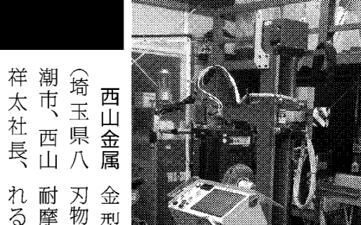
新規導入した「粉体プラズマ自動溶接装置」
