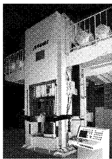
多軸油圧サーボプレス
