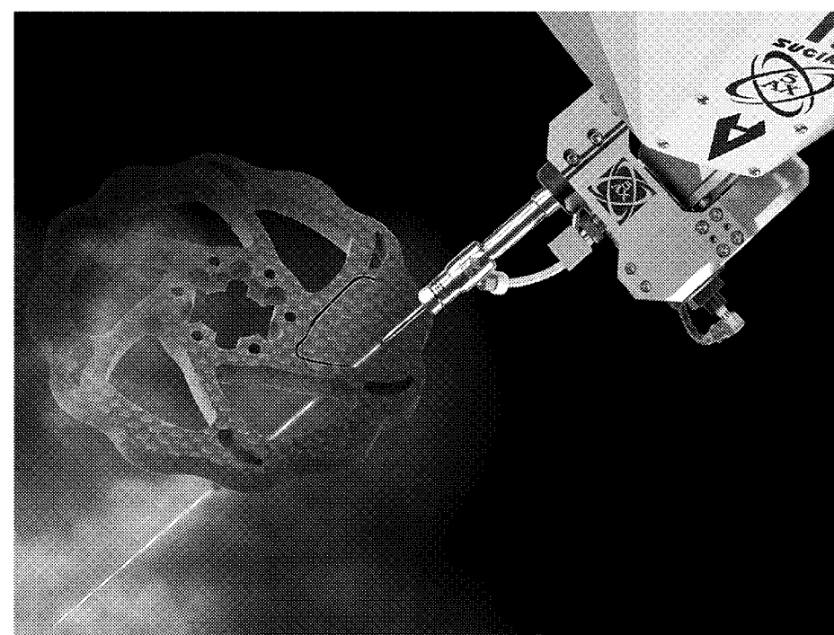
WJ5軸によるCFRP加工
