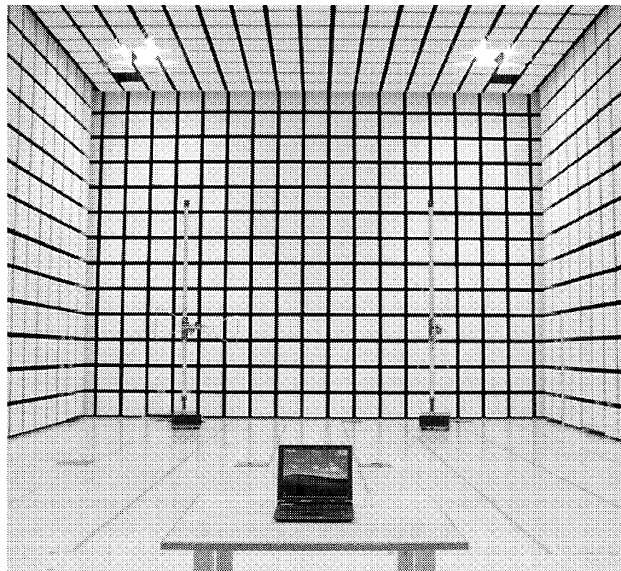
富山県ものづくり研究開発センターの100%法電波暗室
