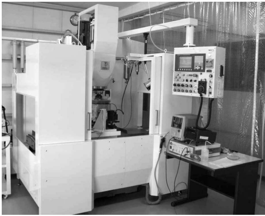
電界トライボケミカル研磨システム実証機
