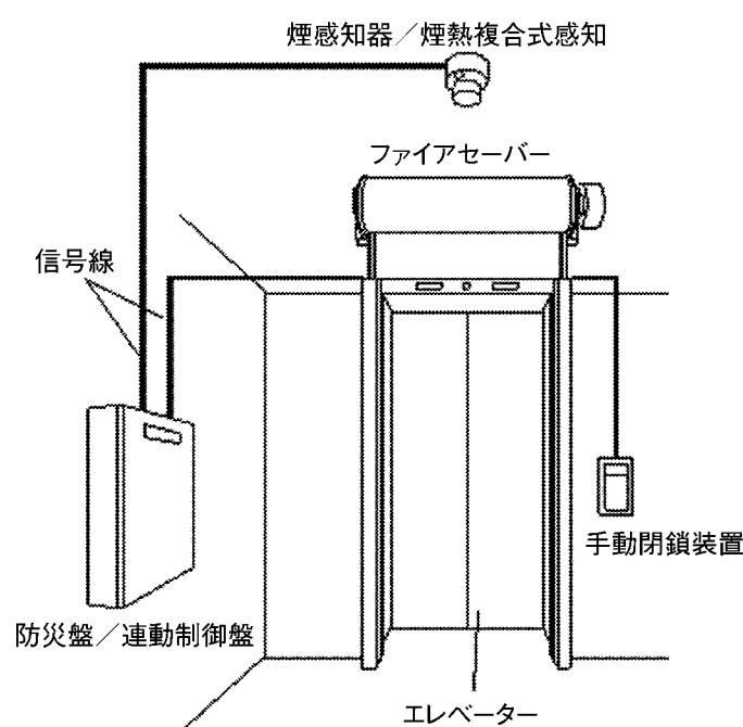
防煙シャッターのシステム図
