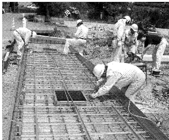
工期を3分の1に短縮したアイ・テックの「ASプレハブ床版橋」
