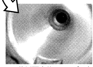
修正研磨後のテーパ穴
